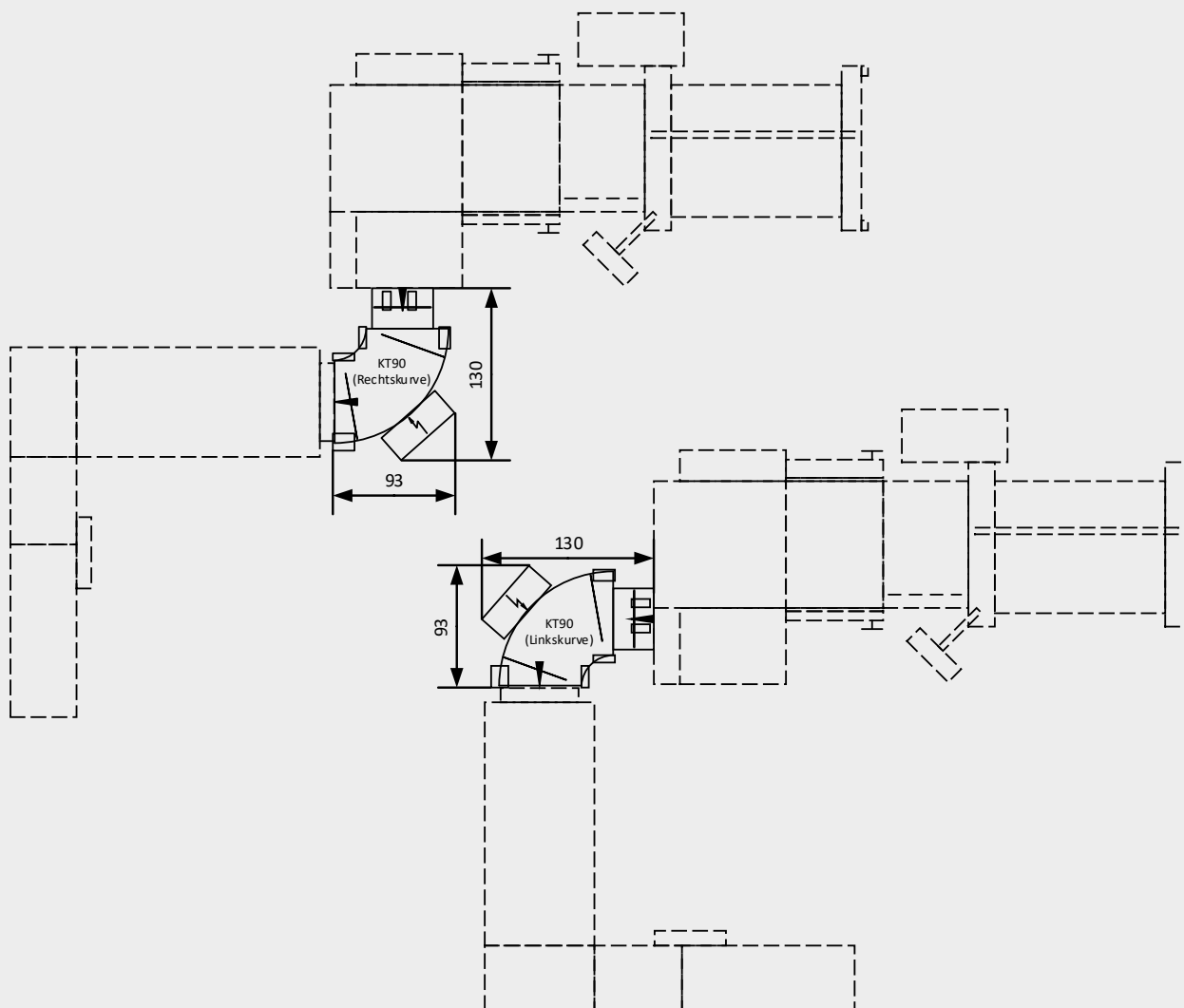
Grundaufbau KT90
