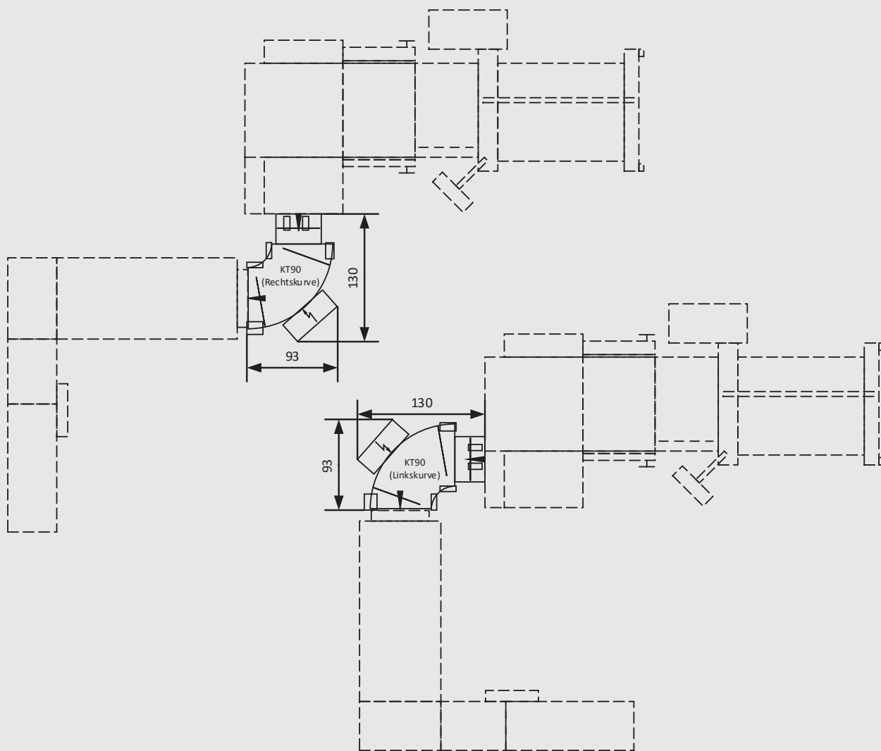
Grundplan
