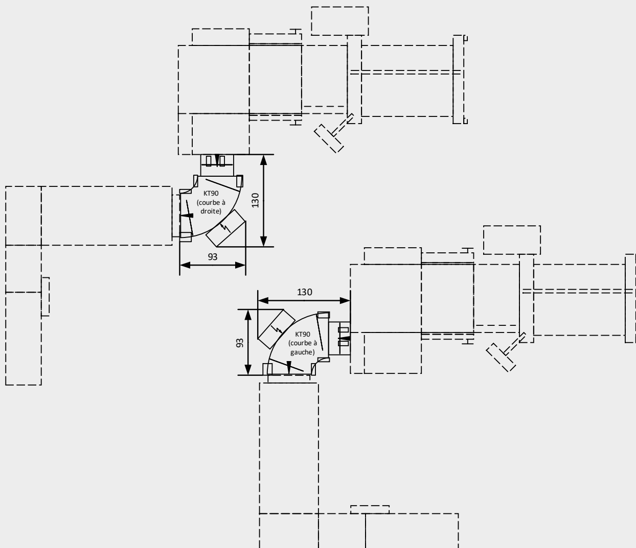
Plan d'implantation KT90
