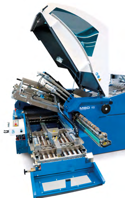
K8 avec cassette à arbres porte-outils amovible et zone ouverte du pli à couteau.
